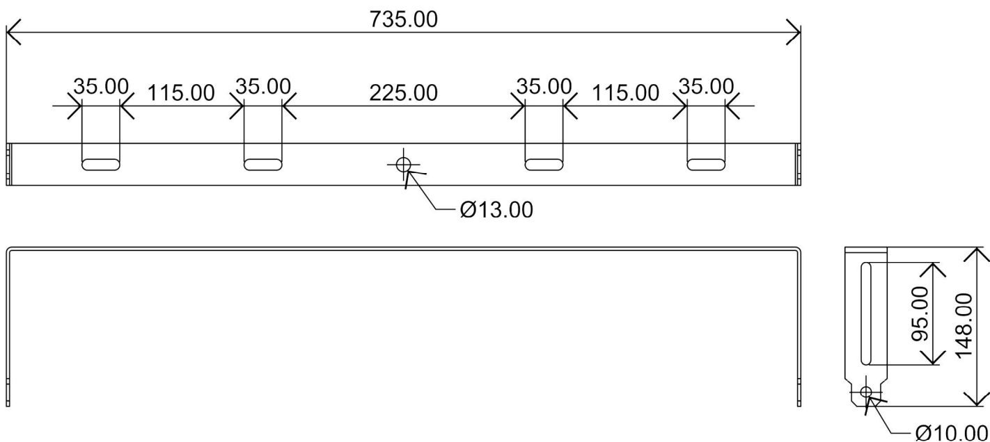
支架 W735mm*L148mm*H50mm 重量0.83KG
