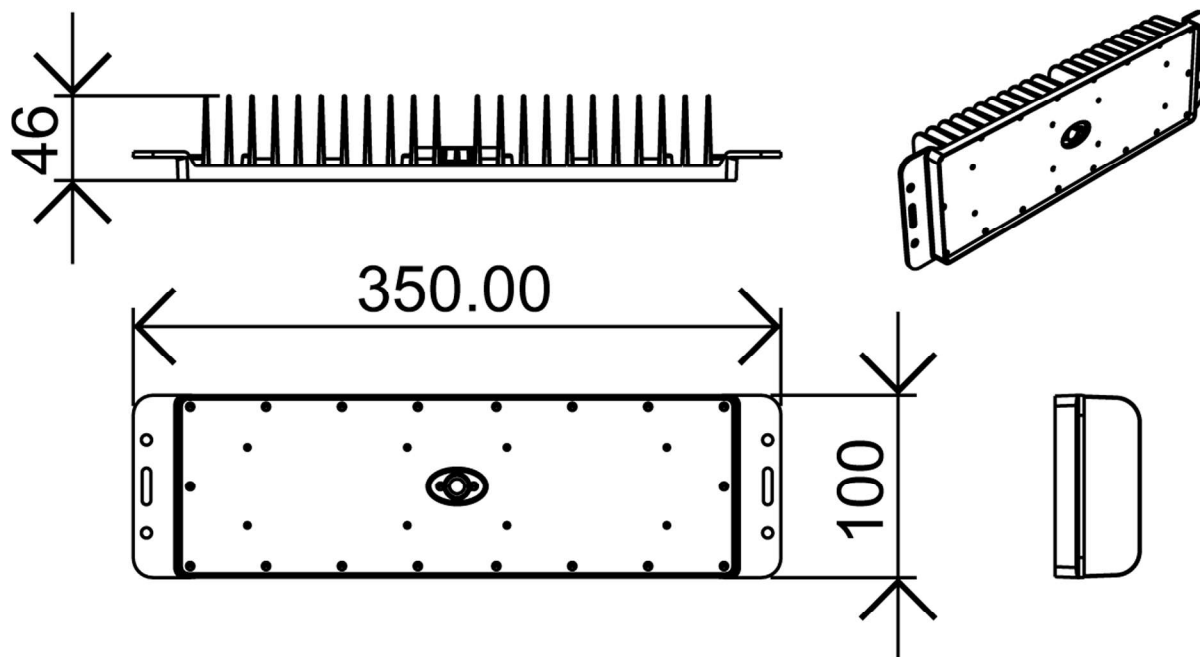
铝合金灯体 W350mm*L100mm*H46mm 重量0.9KG
